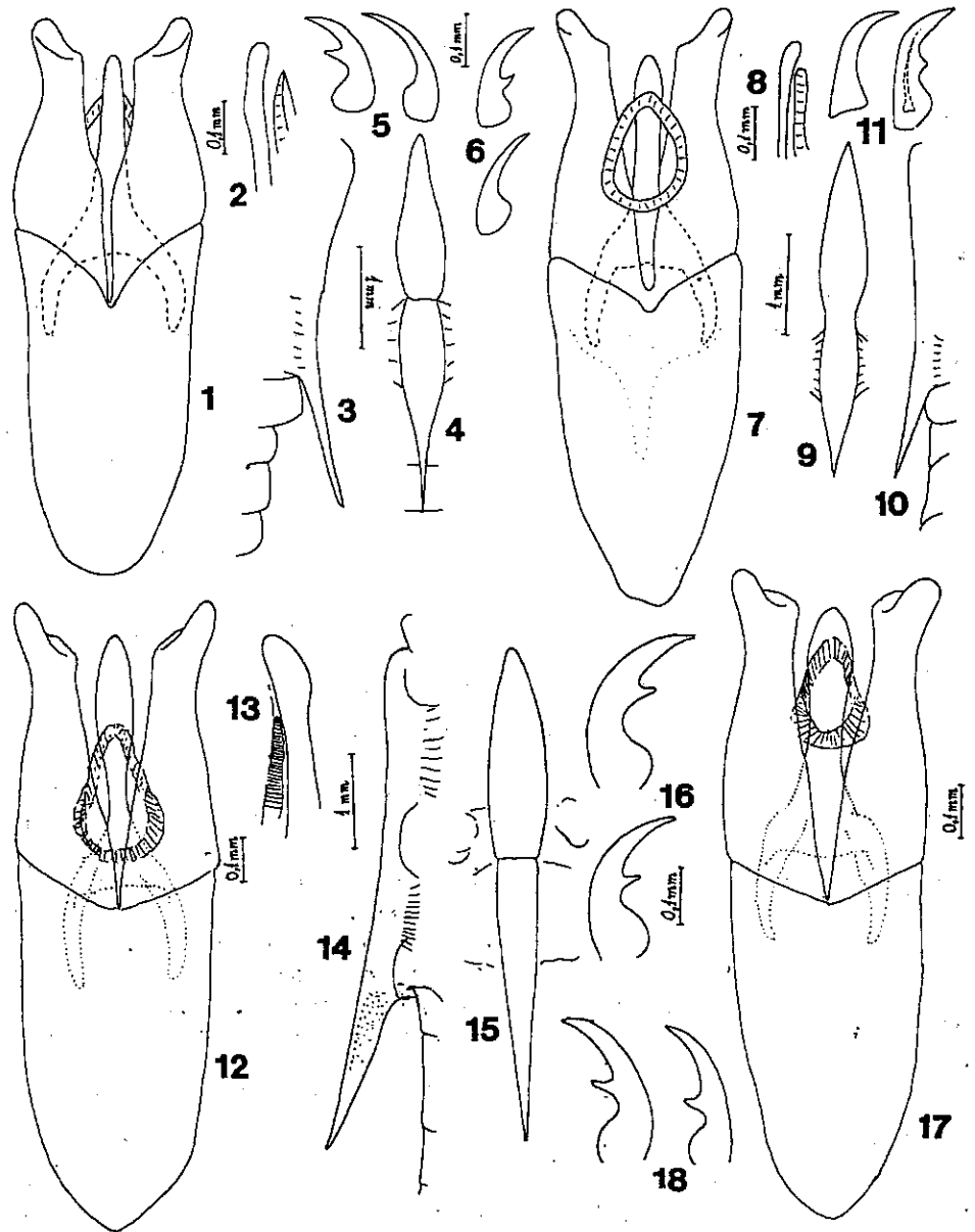
1-6, Tropisternus (Pristoternus) longispina sp. nov.: 1, genitales masculinos, dorsal; 2, extremo del edeago, lateral; 3, carena, lateral; 4, id., ventral; 5, uñas de las patas II del macho; 6, id., de las patas III del macho. 7-11, T. (P.) ignoratus Knisch: 7, genitales masculinos, ventral; 8, extremo del edeago, lateral; 9, carena, ventral; 10, id., lateral; 11, uñas de las patas III del macho. 12-16, T. (P.) burmeisteri sp. nov.: 12, genitales masculinos, ventral; 13, extremo del edeago, lateral; 14, carena, lateral; 15, id., ventral; 16, uñas internas de las patas II y III del macho. 17-18, T. (P.) setiger (Germar): 17, genitales masculinos, ventral; 18, uñas internas de las patas II y III del macho.
